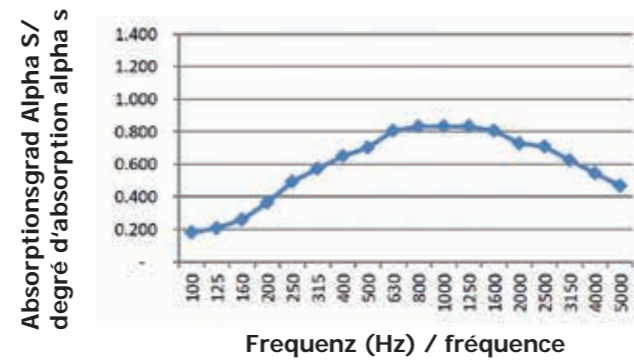
Schallabsorption nach DIN EN ISO 354 coefficient d'absorption selon DIN EN ISO 354
