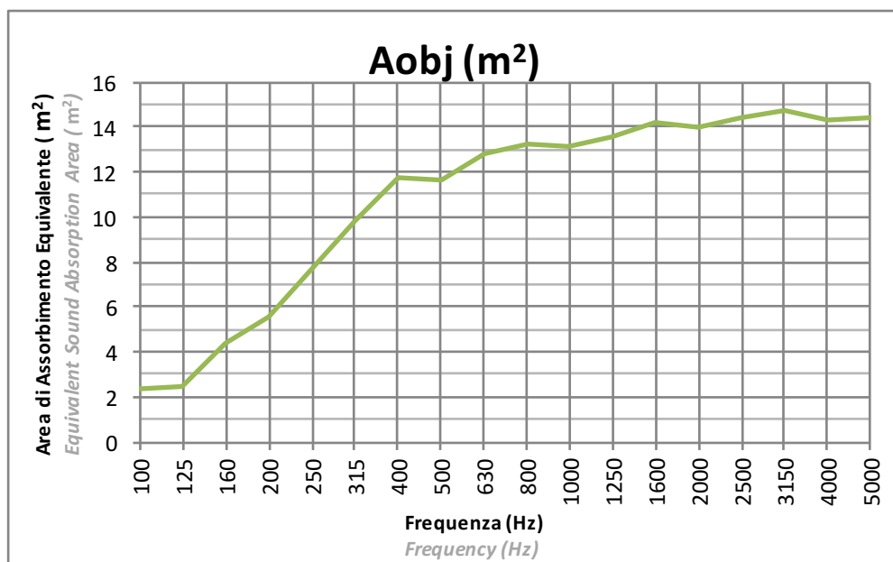
La prova è stata eseguita secondo le prescrizioni della norma UNI EN ISO 354 Test executed according to UNI EN ISO 354
